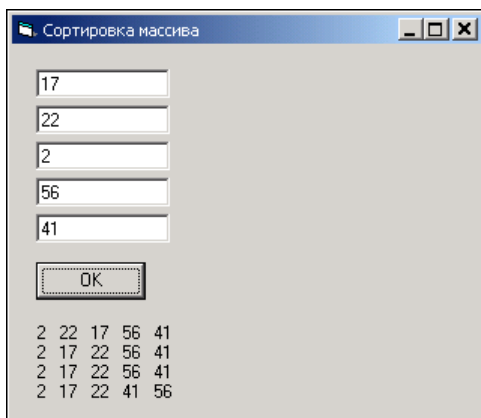
Рис. 3.29. Сортировка массива методом прямого выбора
