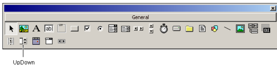
Рис. 9.21. Компонент UpDown
