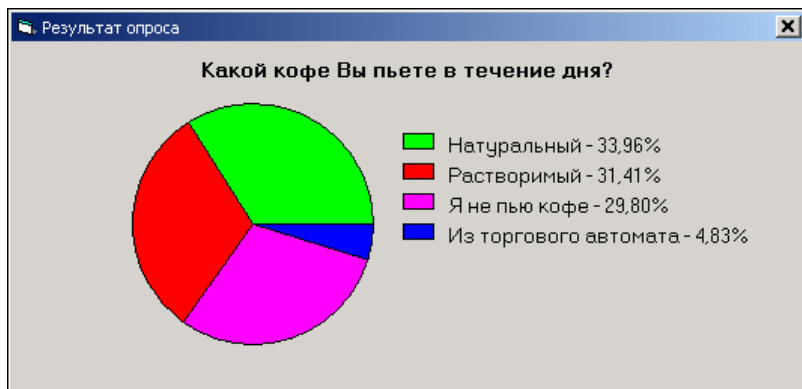
Рис. 5.8. Круговая диаграмма
