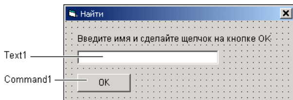
Рис. 7.14. Форма Найти
