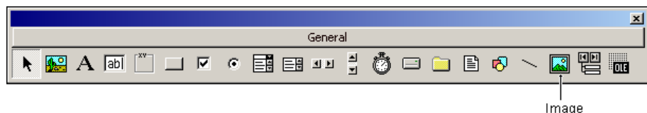
Рис. 4.19. Компонент Image
