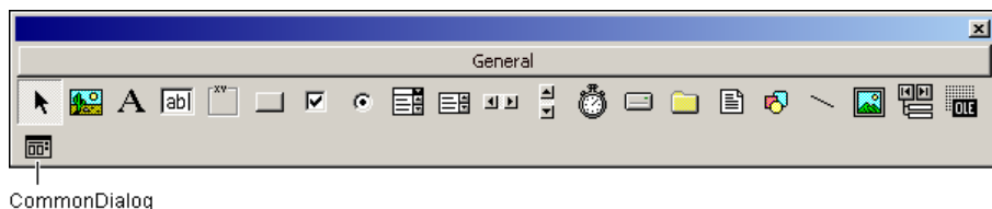
Рис. 9.4. Компонент CommonDialog
